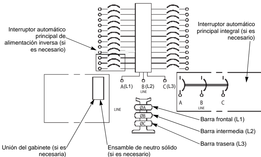
Figura 6: Diagrama de alambrado del interruptor automático principal / zapatas principales
