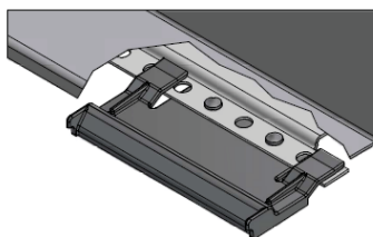
Extensión de relleno HLN4EBL en el lado angosto
